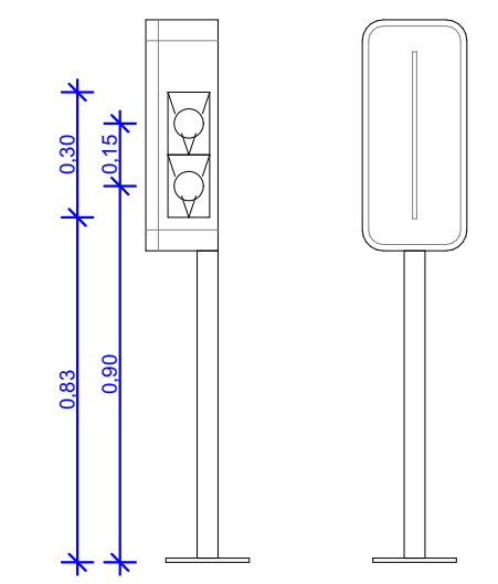
Détail Borne de recharge 1:20
